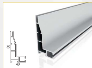
EF - LS80
