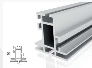
EF - FD40
