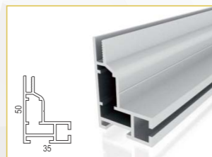
EF - LS50
