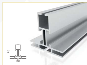
EF - FD50
